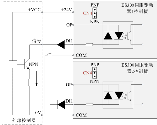
图3-10. 多台伺服驱动器DI端子并接漏型接线方式
