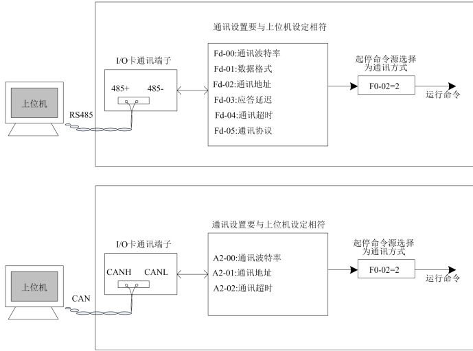
图4-7. 通讯控制启停示意图
