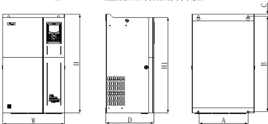
图 2-4. 30~37kW 钣金机箱外形尺寸及安装尺寸示意图
