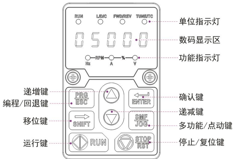
图4-1. 操作面板示意图
